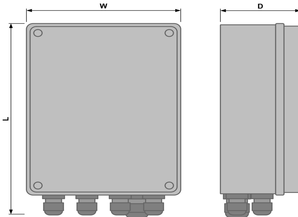
Ogólny widok urządzenia
