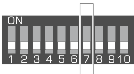
Rys. 4. Przełącznik do włączenia / wyłączenia obsługi niezarejestrowanego testera ARF-200.
